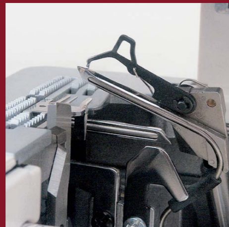
Griffe très puissante avec griffe auxiliaire orientable
